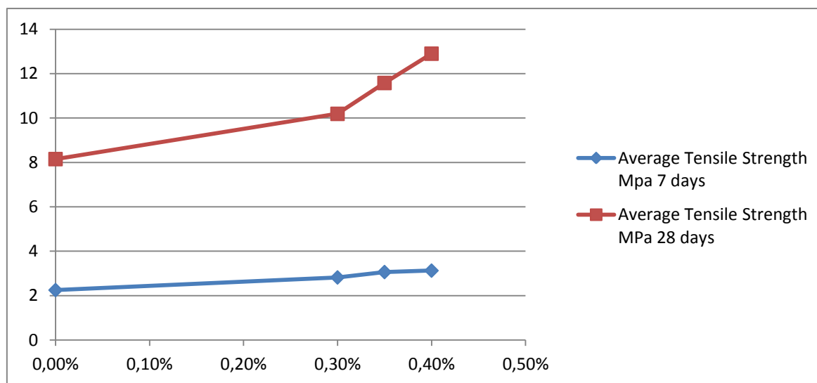
Tensile strength (MPa)
